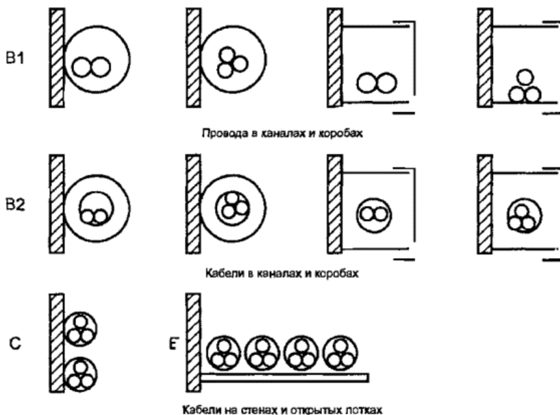
Рисунок С.1 - Методы укладки кабелей и проводов
