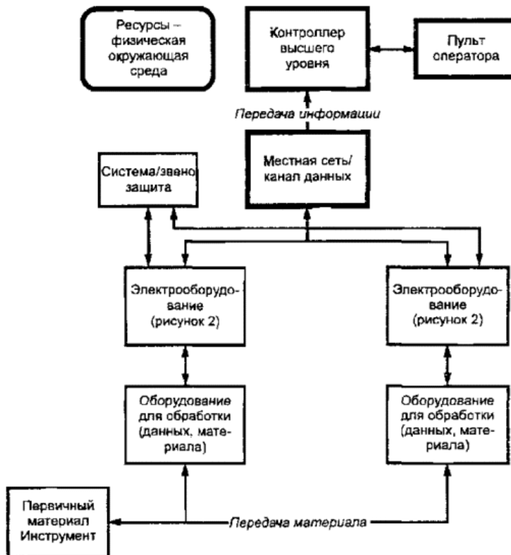
Рисунок 1 - Функциональная схема типовой производственной системы
