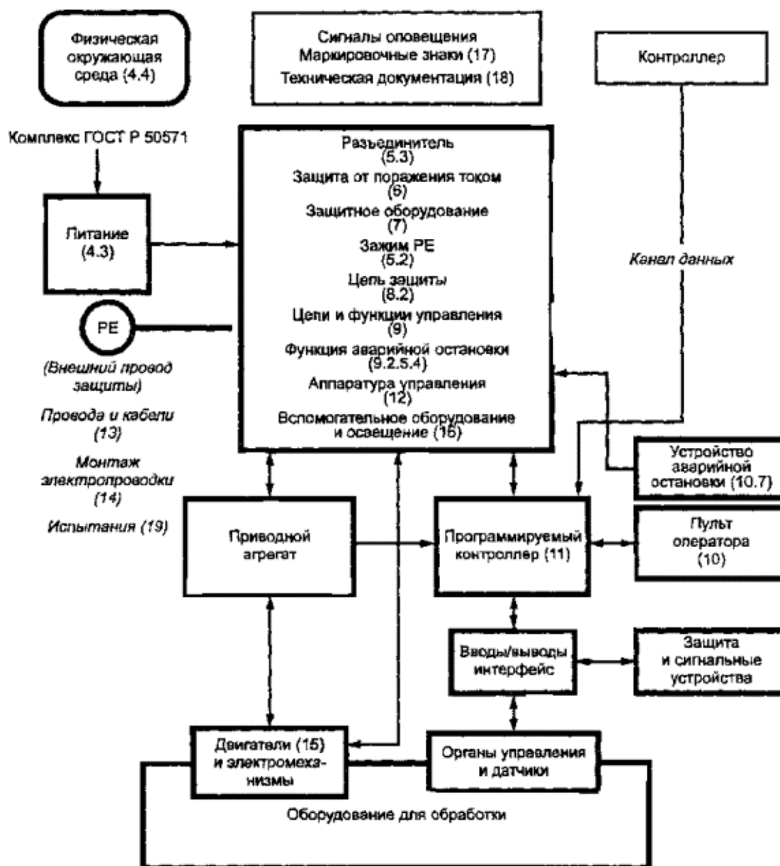
Рисунок 2 - Функциональная схема типовой машины
