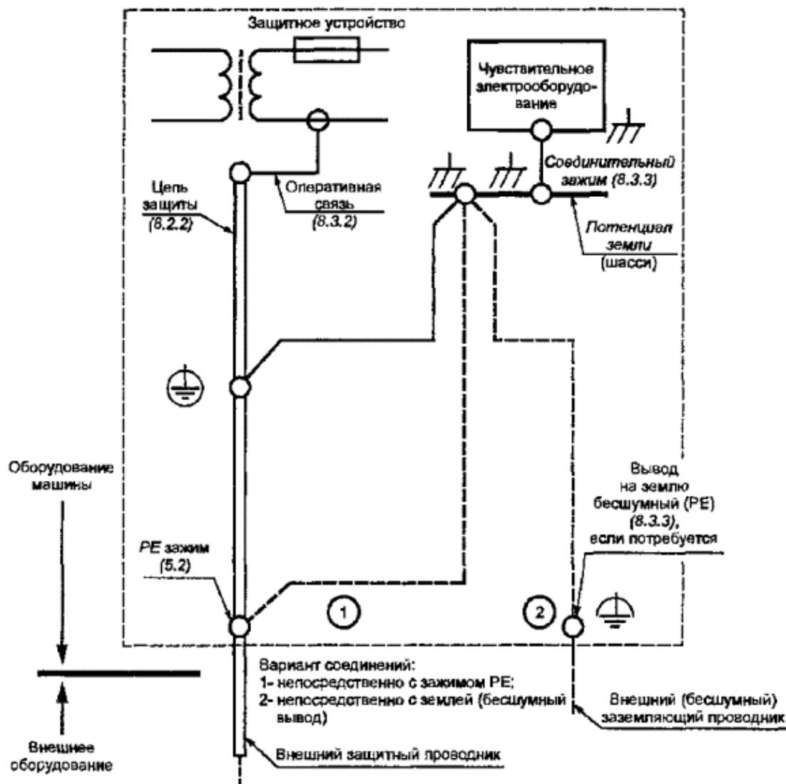
Рисунок 3 - Пример эквипотенциального соединения машины
