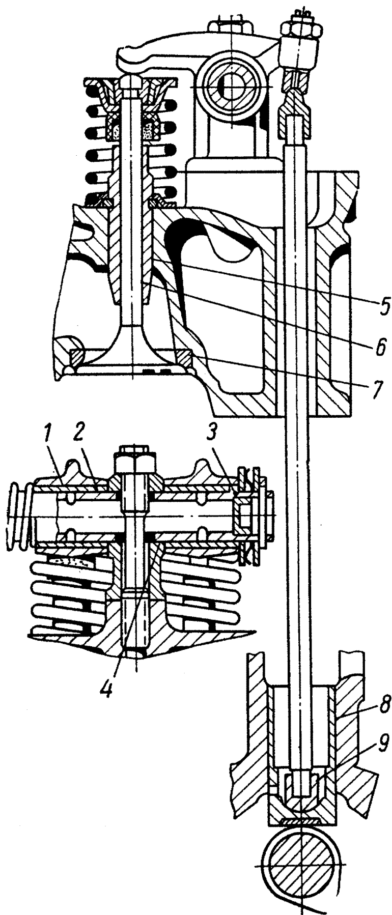
Рис. 238 Газораспределительный механизм
