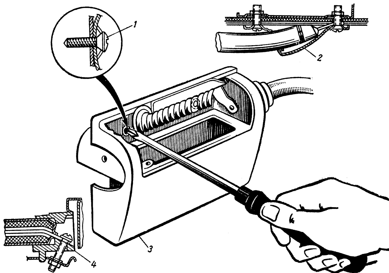
Рис. 151. Демонтаж пепельницы:
