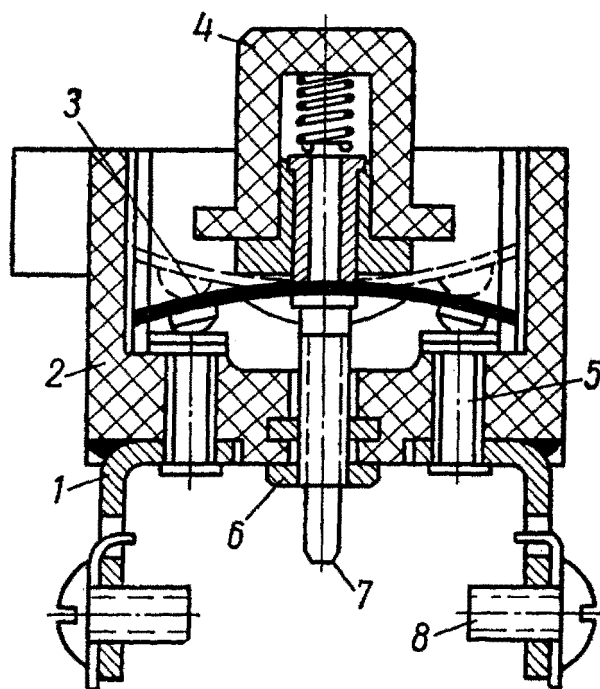
Рис. 224. Биметаллический предохранитель:
