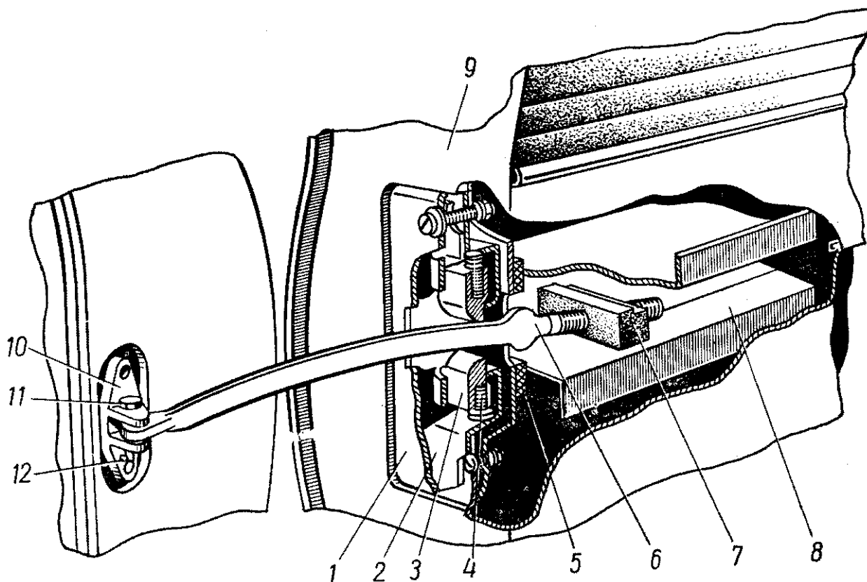
Рис. 147. Ограничитель двери:
