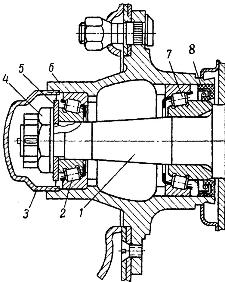
Рис. 120 Ступица переднего колеса:
