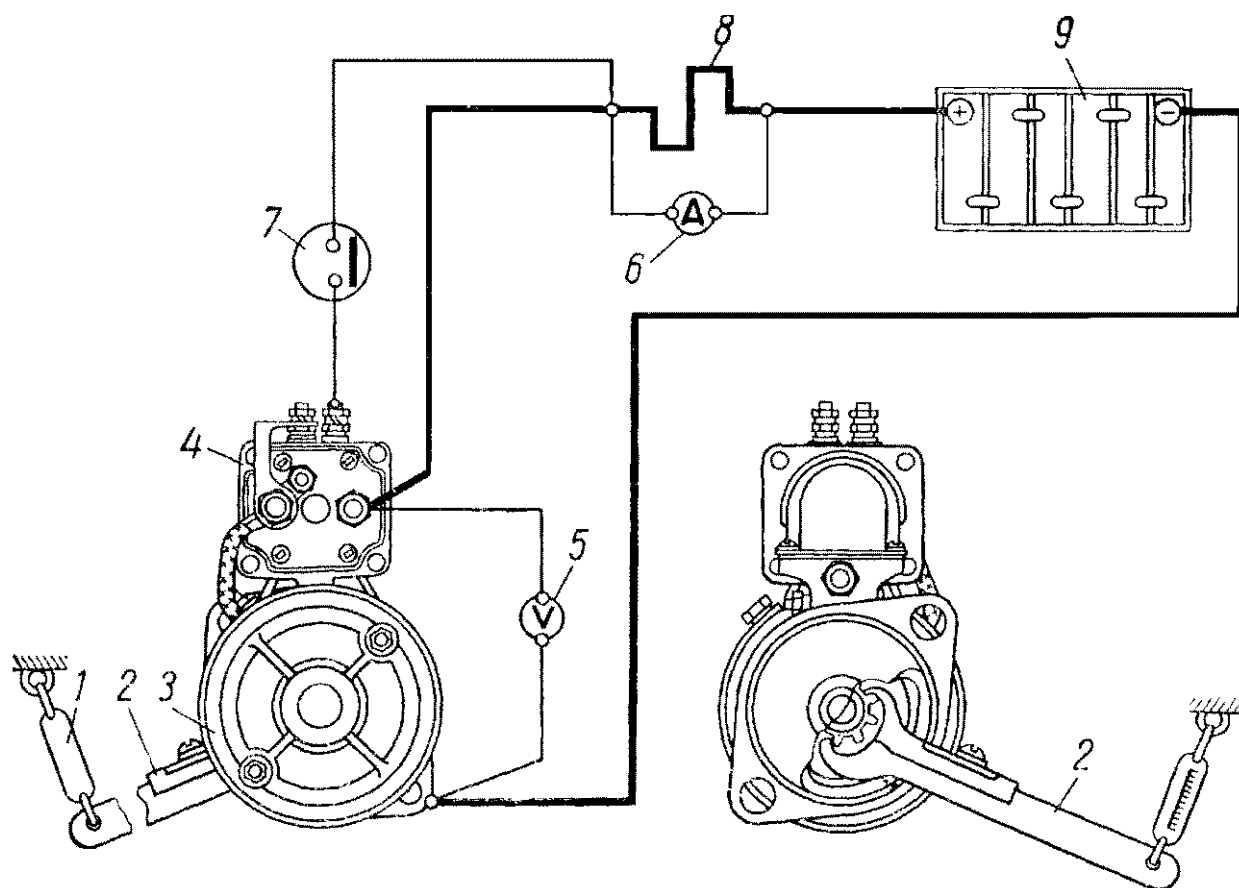
Рис. 190. Схема включения стартера для проверки:
