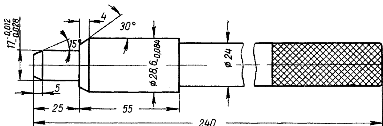
Рис. 83. Оправка для установки ведомого диска сцепления
