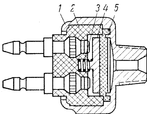
Рис. 203. Включатель стоп-сигнала:
