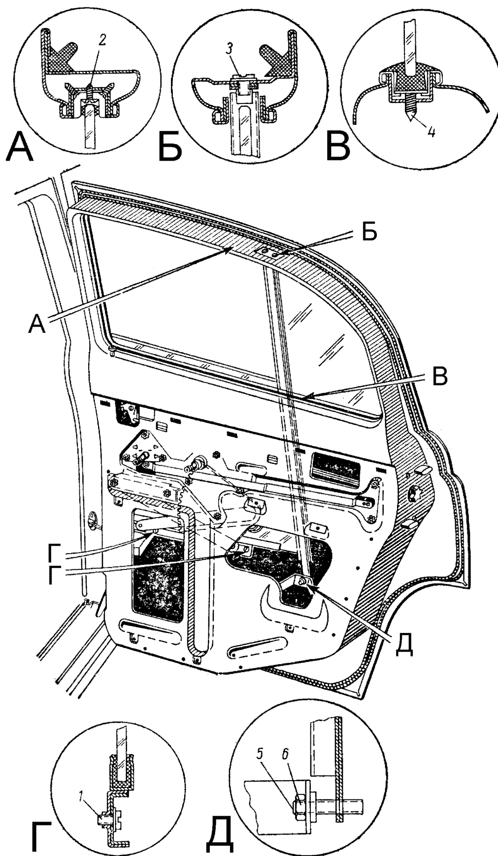
Рис. 153. Задняя дверь:
