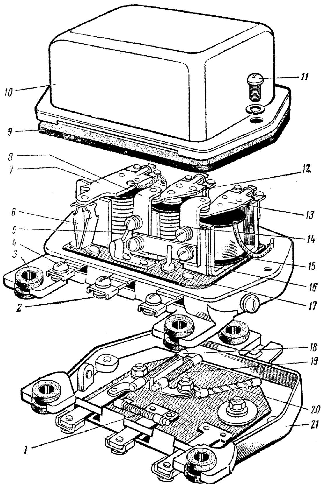
Рис. 180. Реле-регулятор:
