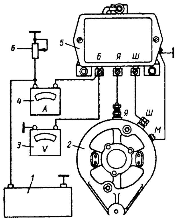
Рис. 183. Схема включения приборов для проверки регулятора напряжения и ограничителя силы тока:
