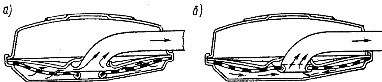
Рис. 14. Схема работы маслоприемника: а — при незасоренной сетке; б — при засоренной сетке
