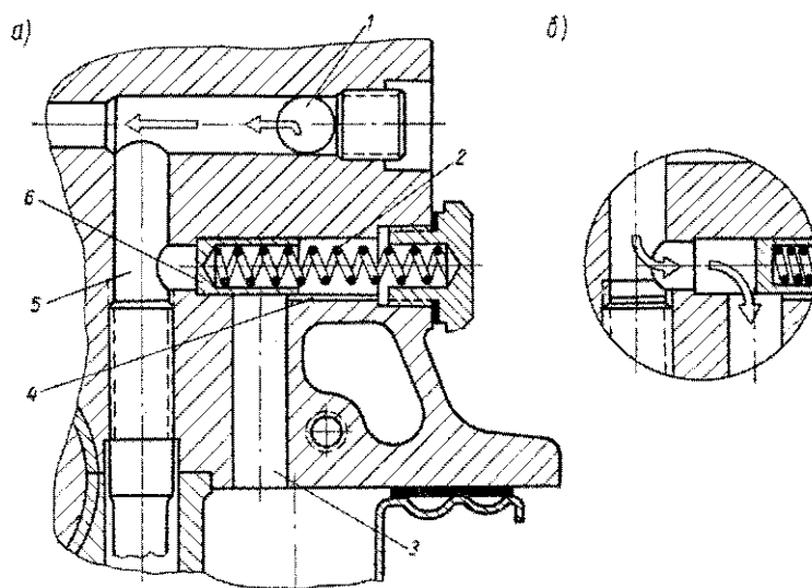
Рис. 17. Схема подвода масла к редукционному клапану: а — редукционный клапан закрыт; б — редукционный клапан открыт;
