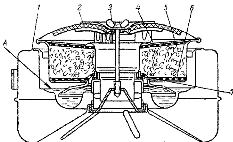
Рис. 49. Воздушный фильтр
