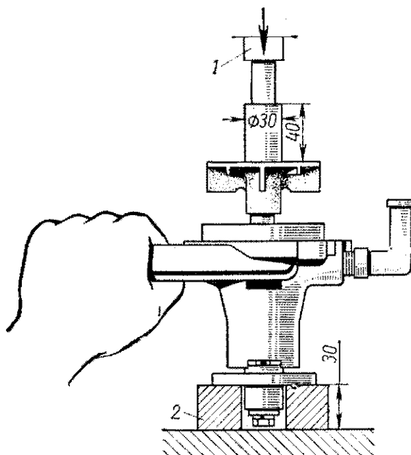
▲ Рис. 35. Напрессовка крыльчатки водяного насоса:
