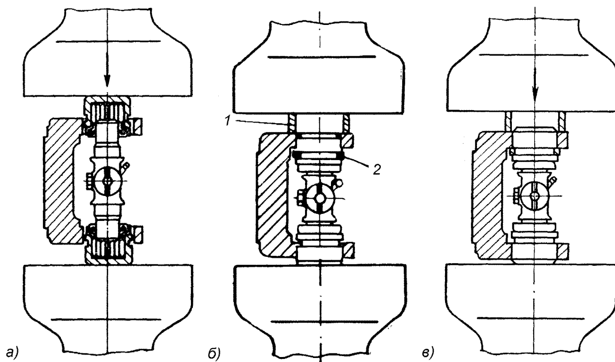
Рис. 102. Сборка кардана:
