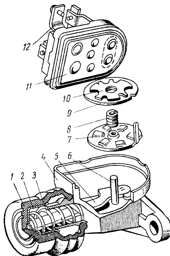
Рис. 202. Ножной переключатель света:
