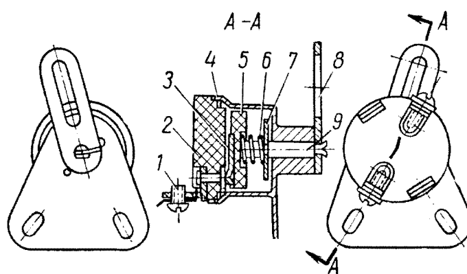
Рис. 204. Включатель света заднего хода:
