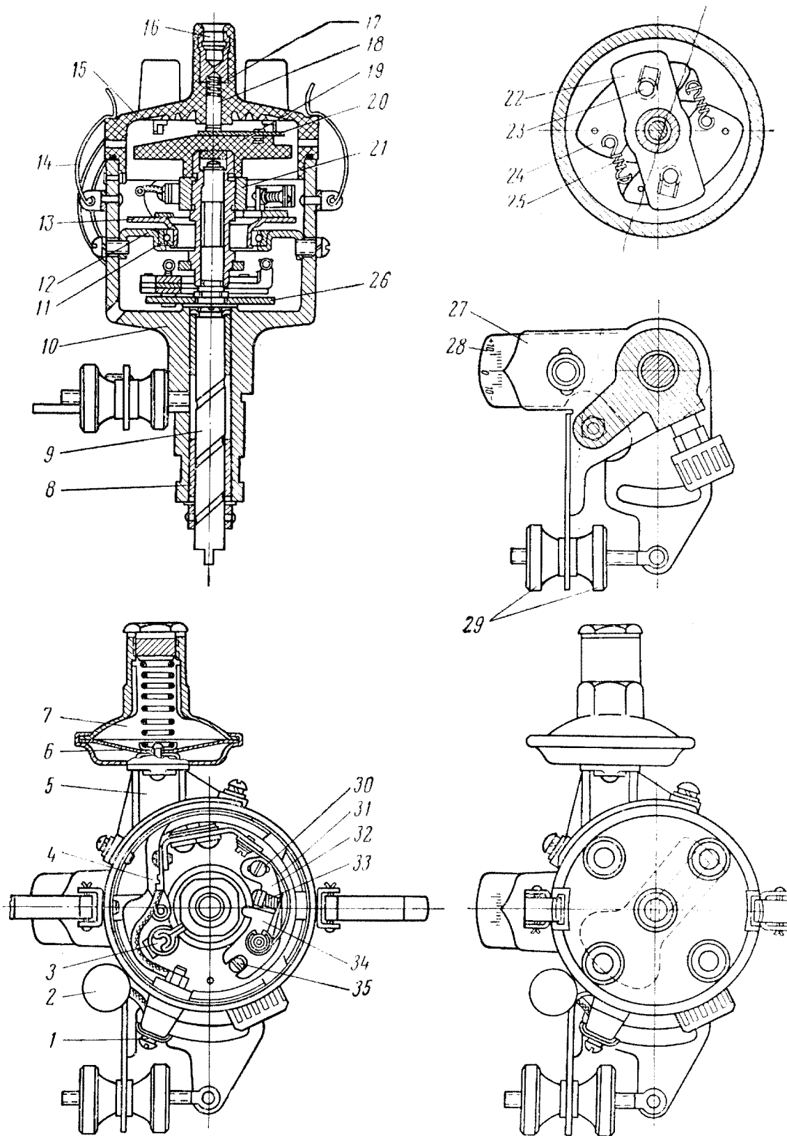
Рис. 194. Прерыватель-распределитель:
