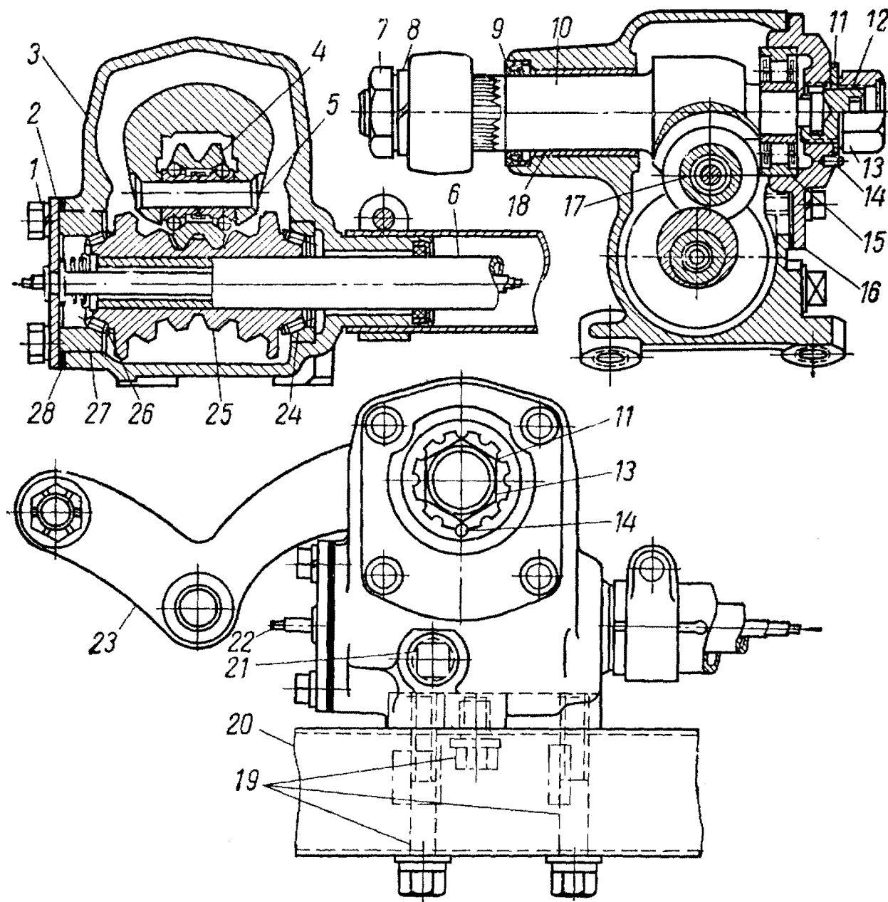
Рис. 158. Рулевой механизм:
