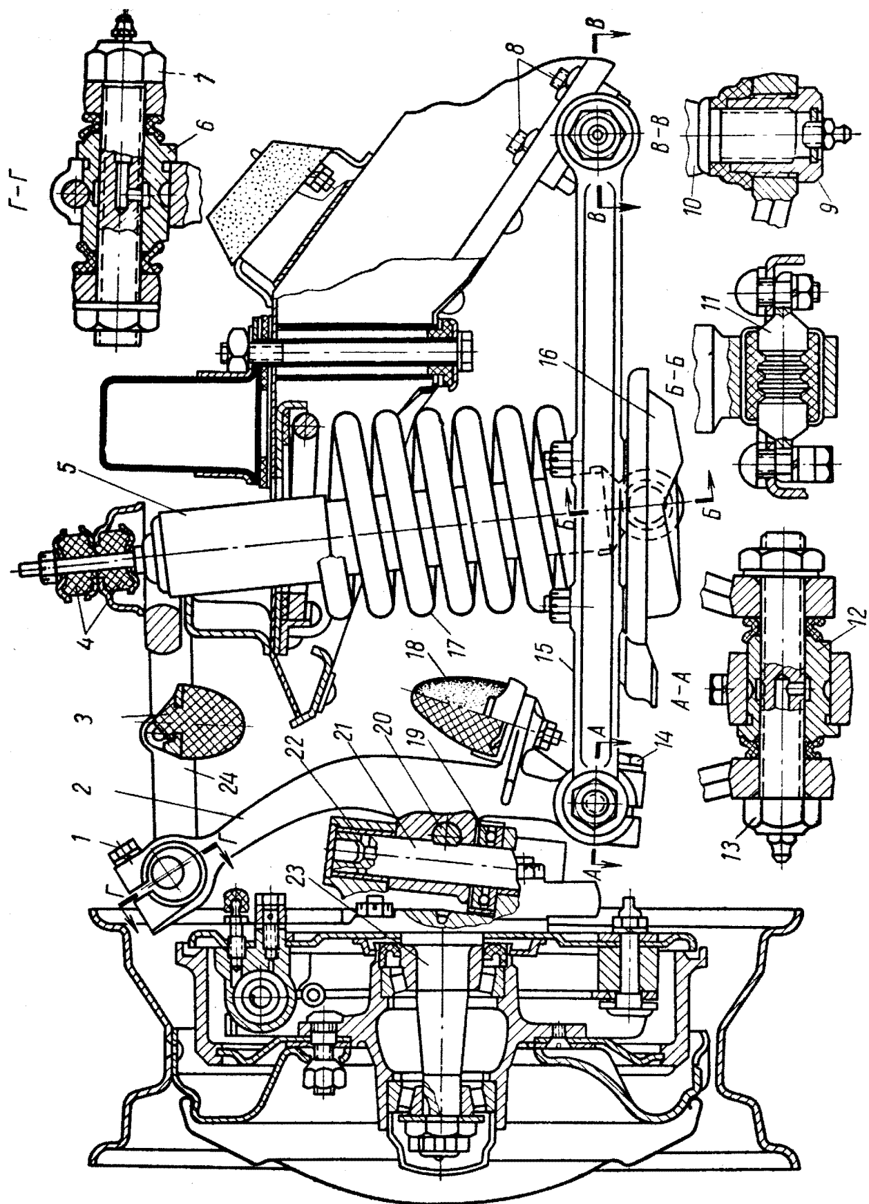
Рис. 119. Передняя подвеска:
