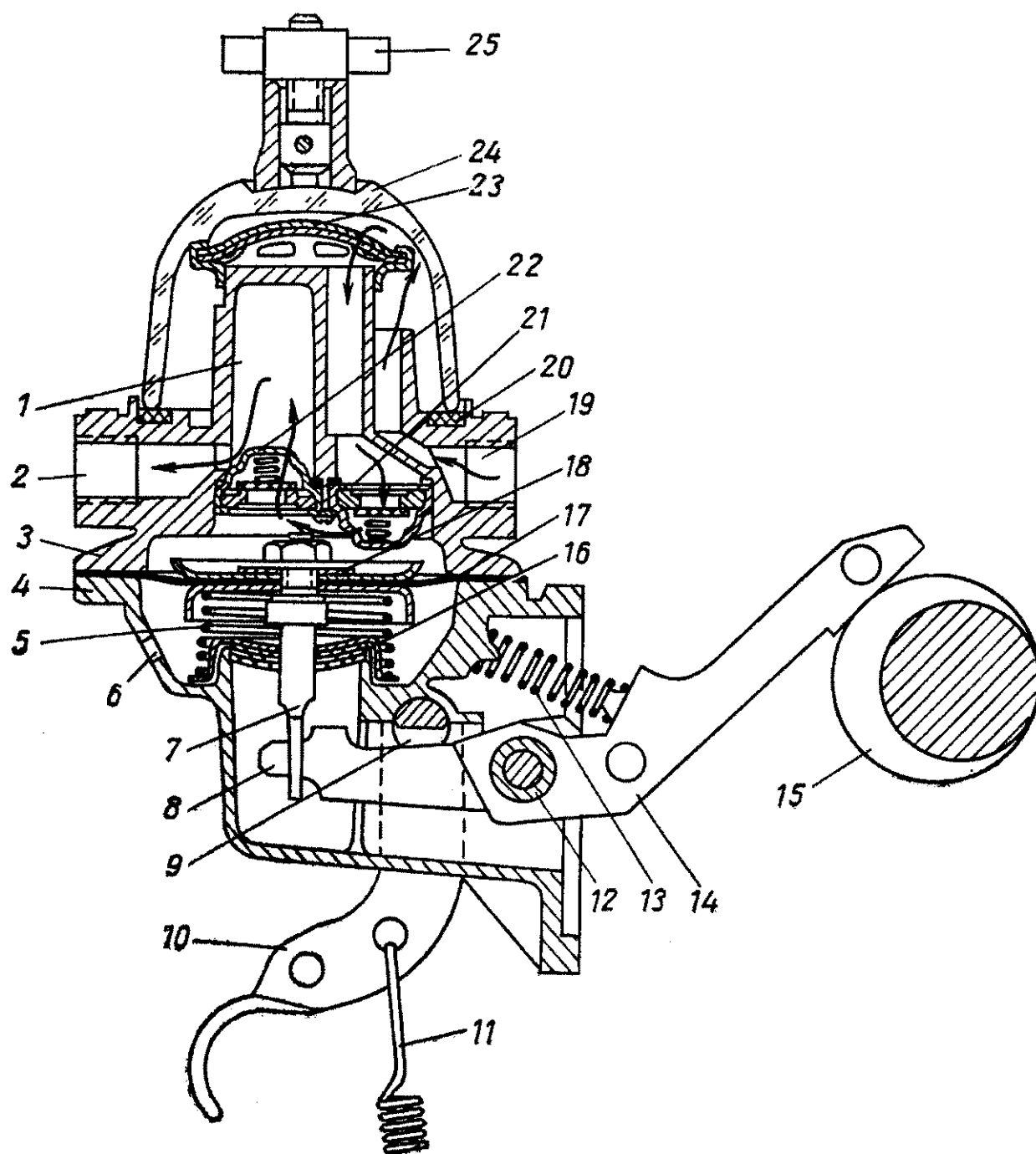
Рис. 43. Топливный насос:
