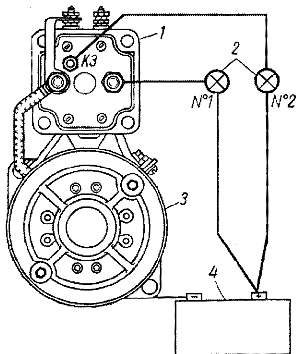
Рис. 188. Схема проверки регулировки включателя стартера:
