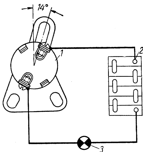
Рис. 215. Схема проверки включателя света заднего хода:
