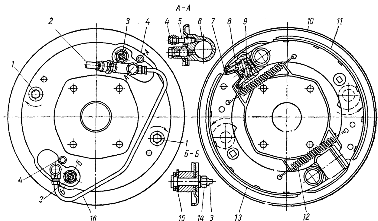
Рис. 164. Передний тормоз:
