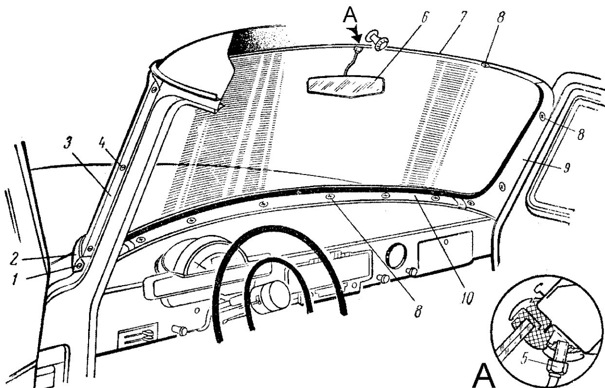
Рис. 154. Ветровое окно:
