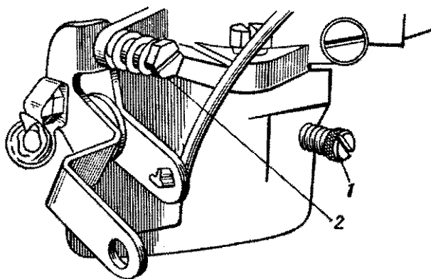
Рис. 53. Регулировочные винты карбюраторов
