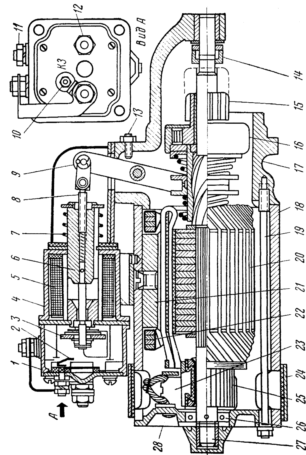
Рис. 185. Стартер:
