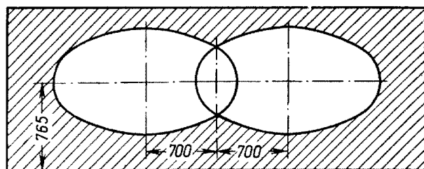
Рис. 209. Экран для регулировки фар
