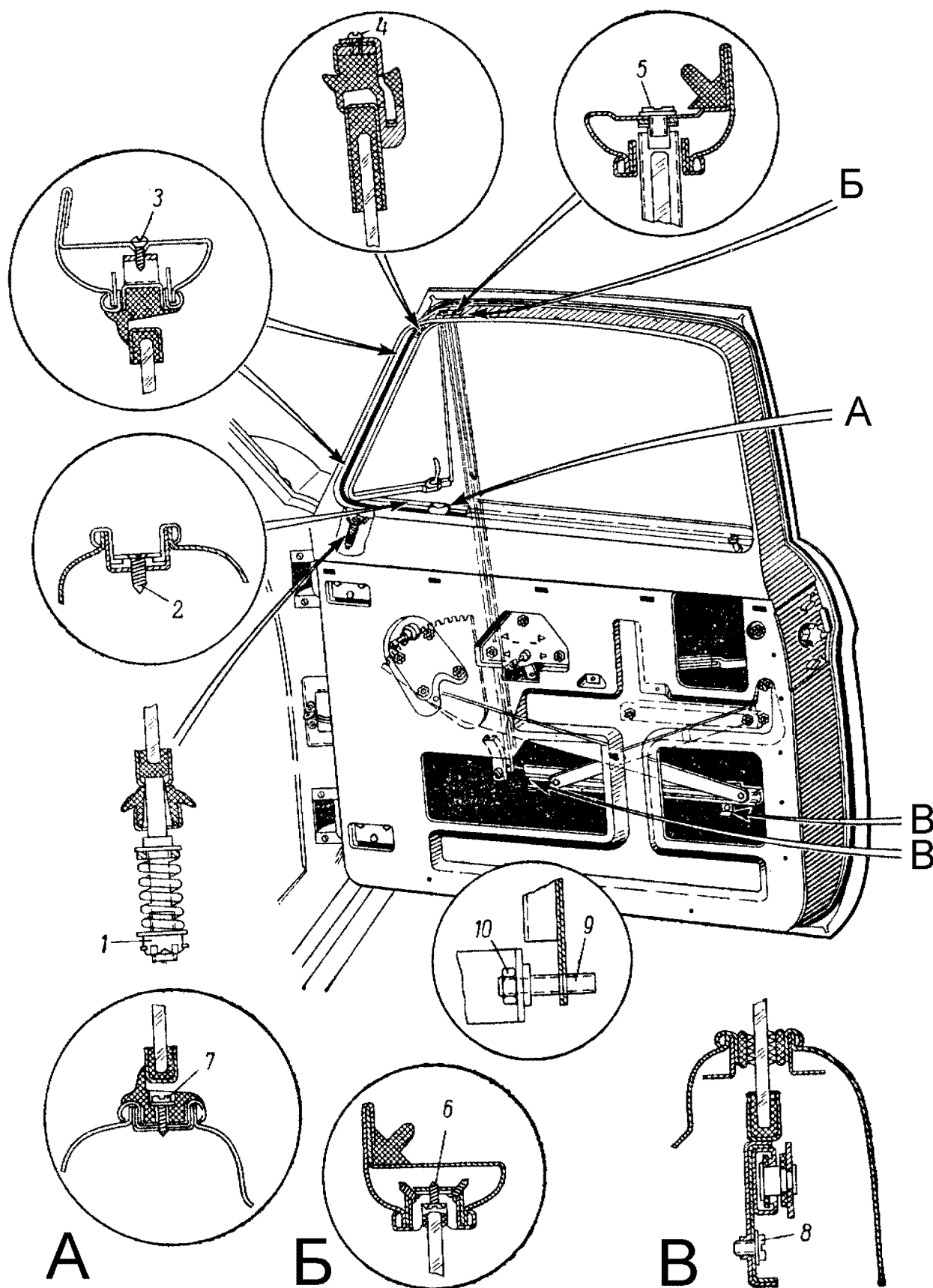
Рис. 152. Передняя дверь:
