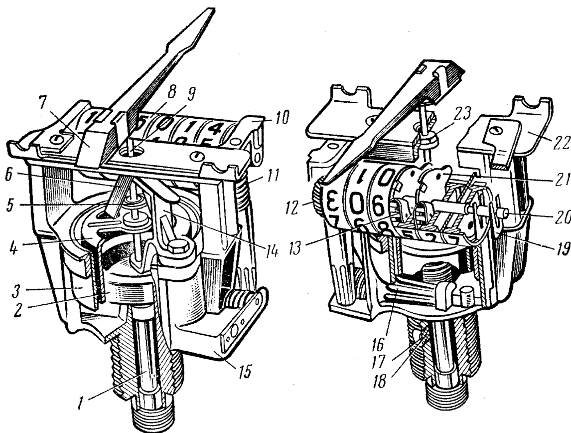
Рис. 226. Механизм спидометра:
