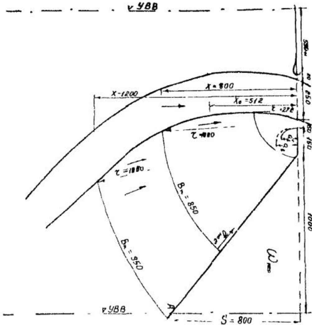
Рис. 12. План участка реки в районе мостового перехода
