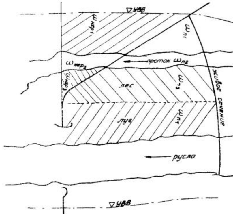
Рис. 7. Схема к определению продольного стеснения поймы
