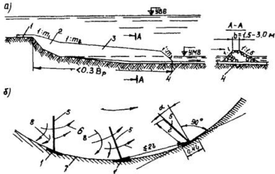
Рис. 14. Схема защиты размываемого берега полузапрудями:
