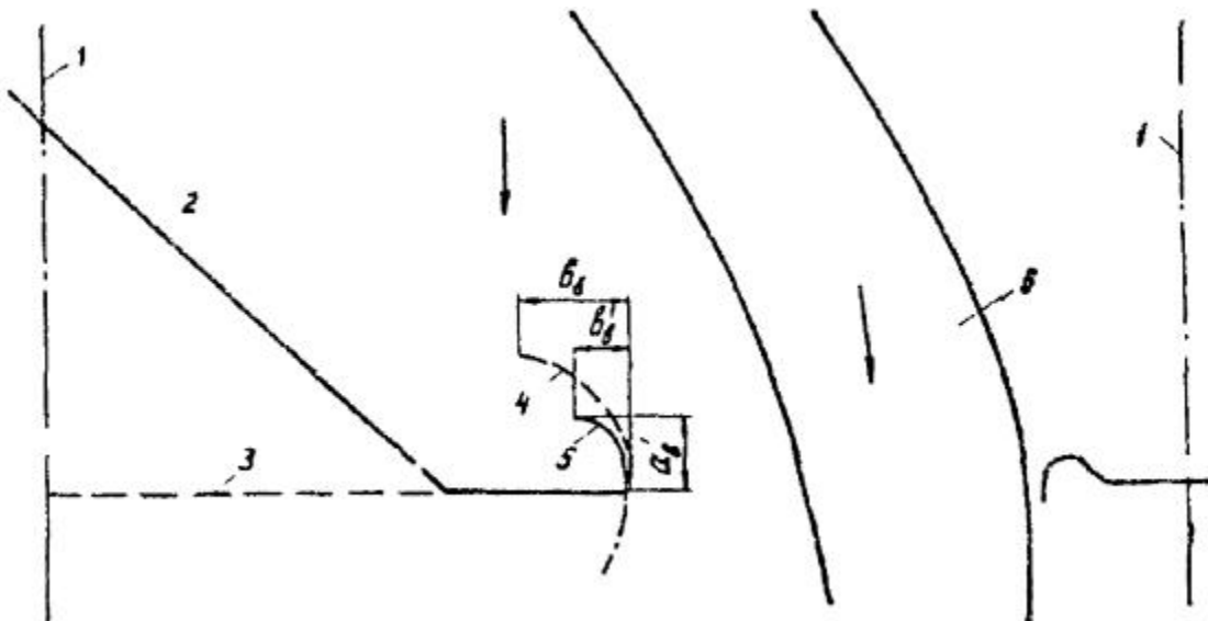
Рис. 5. Параметры струенаправляющих дамб:
