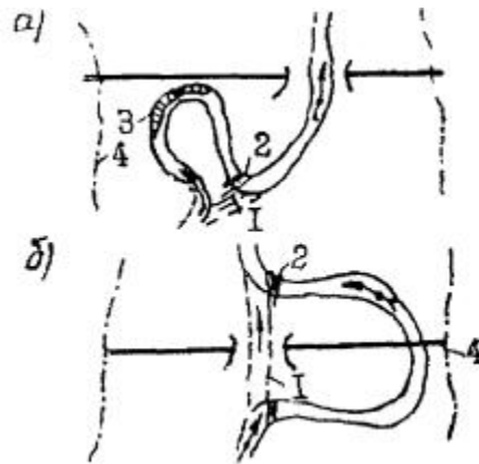
Рис. 13. Схема спрямлений излучен русла:
