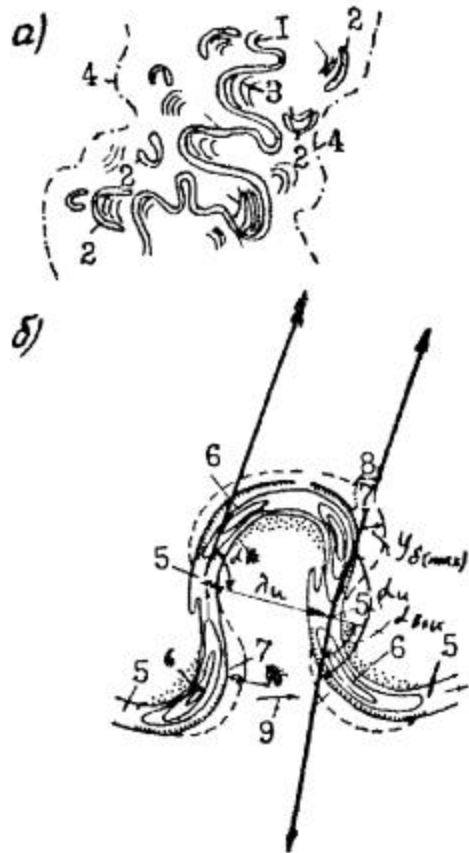
Рис. 1. План свободно меандрирующего русла:
