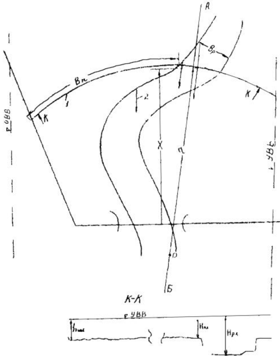
Рис. 10. Нанесение пойменного живого сечения на план участка:
