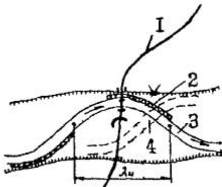
Рис. 3. Схема перехода через реку с ограниченно меандрирующим руслом:
