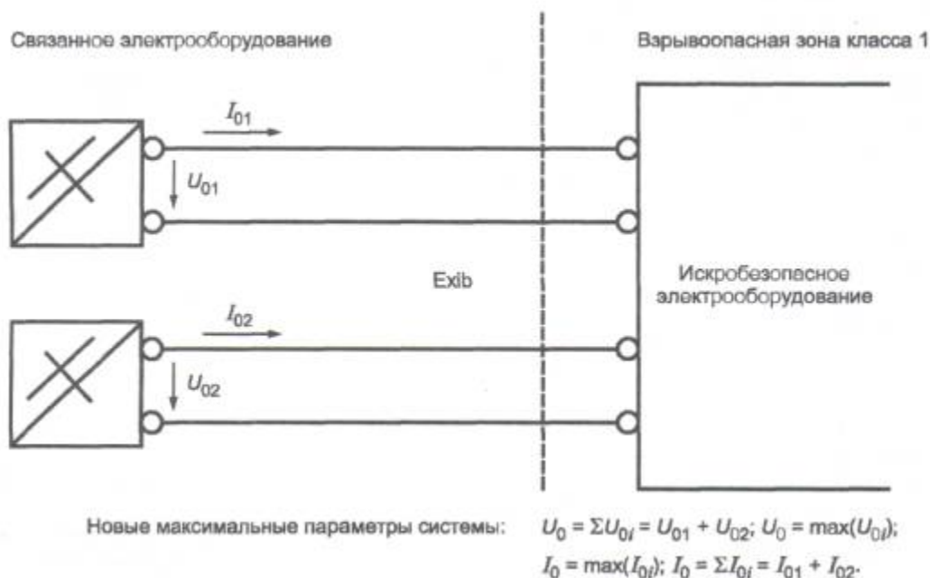
Рисунок В.3 - Последовательные и параллельные соединения. Суммирование напряжений и токов
