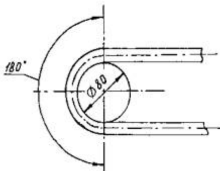
Рисунок 5 - Схема определения работоспособности воздуховодного шланга
