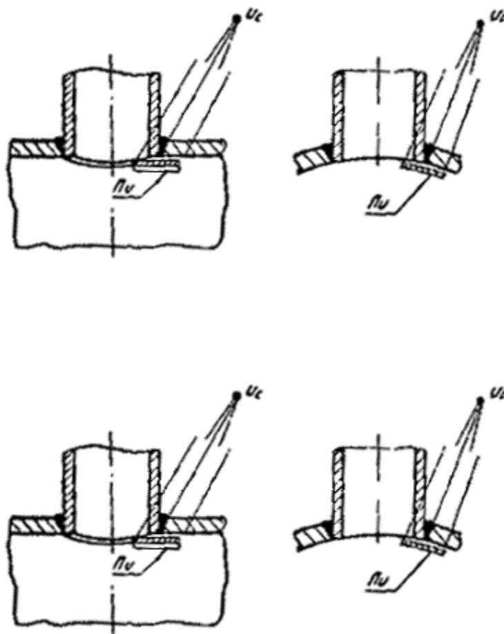
Рис. 10. Схемы просвечивания криволинейных швов врезок снаружи трубы за несколько установок источника излучения
