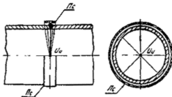
Рис. 3. Схема фронтального просвечивания через две стенки за три установки источника излучения
