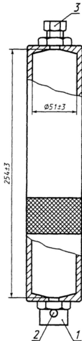
Жидкостная камера с двумя отверстиями
