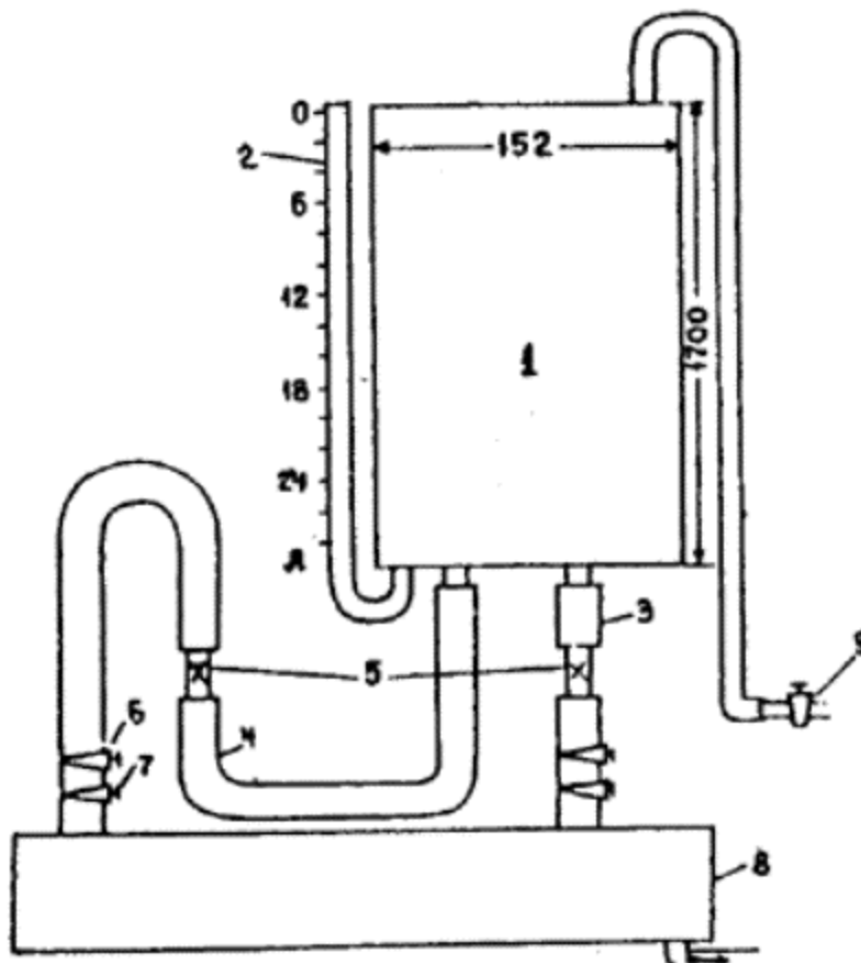
Стенд для тарировки глубинного расходомера
