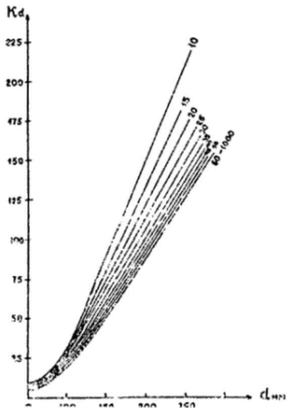
График поправочных коэффициентов за диаметр скважины для расходомера ТСР-34 .
