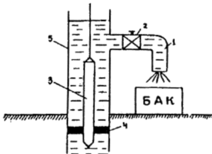
Схема для тарировки расходомеров
