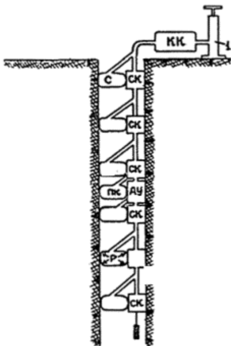
Рис 1. Схематическая конструкция сейсмического зонда.
