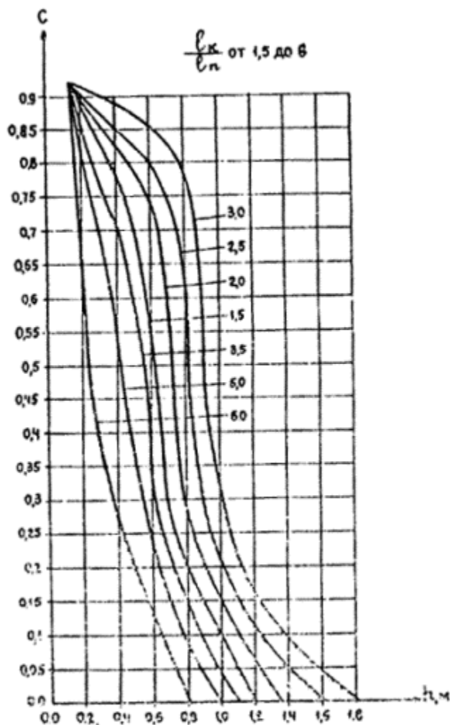
Палетка кривых C = f(h)
